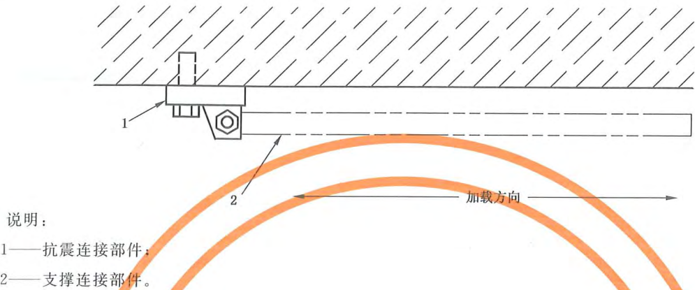
图 1 抗震连接部件加载示意图
