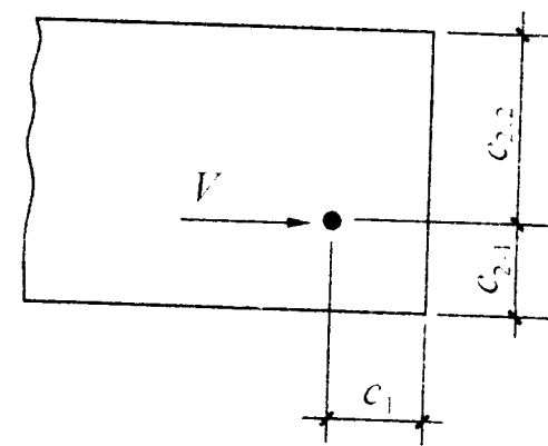
图 6.2.21 有多个边缘影响的锚栓示意
