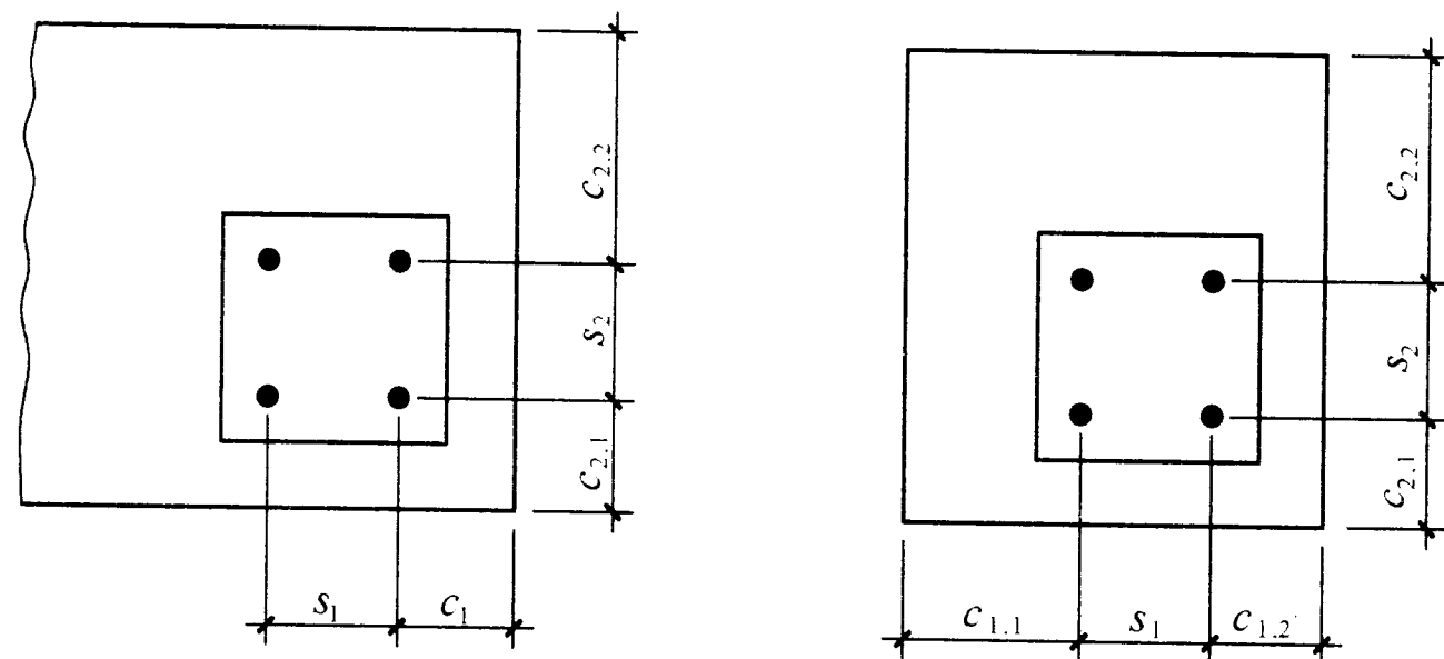
(a) 三个边缘
