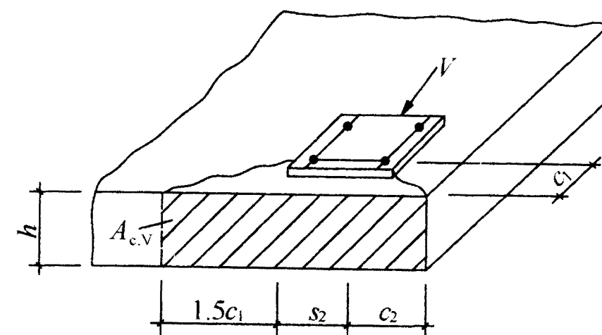
图 6.1.18-3 四栓受剪，位于构件角部示意
