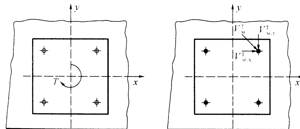
图 5.3.5 扭矩作用下锚栓受剪示意
