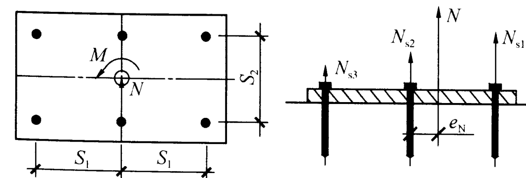
图 5.2.4-1 第一种情况的群锚单向偏心受拉示意
