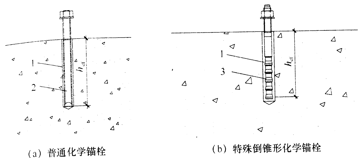
图 A.1.4 化学锚栓示意
