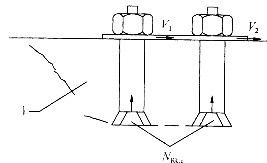
图 6.1.26 锚栓剪撬破坏示意
