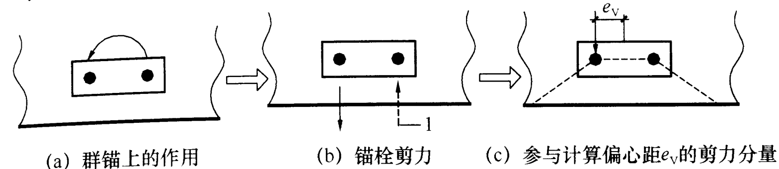
图 5.3.8-1 仅有扭矩作用示意
