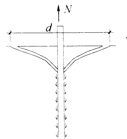
图 A. 2. 3 混合型受拉破坏示意
