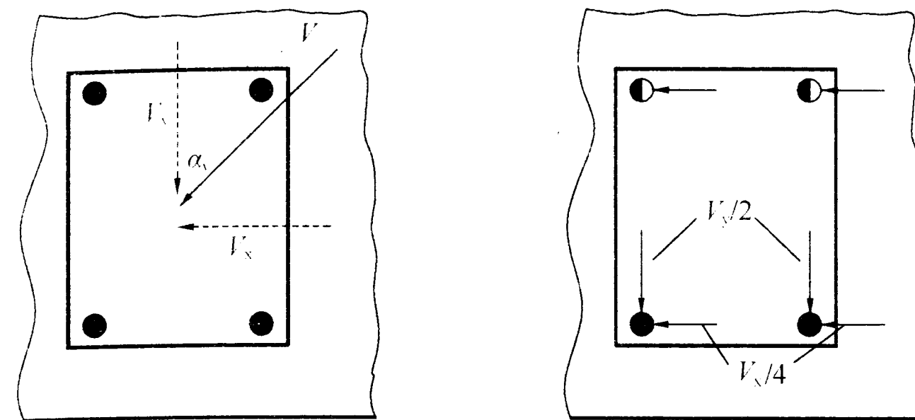
(a) 作用在群锚上的剪切荷载示意
