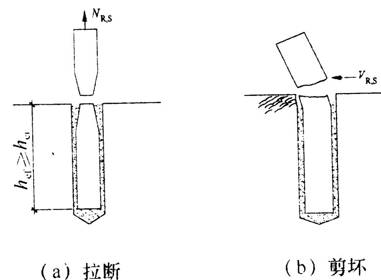
图 A.2.1 锚固钢材破坏示意
