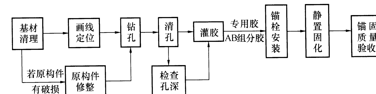
图 5 化学锚栓施工工序示意
