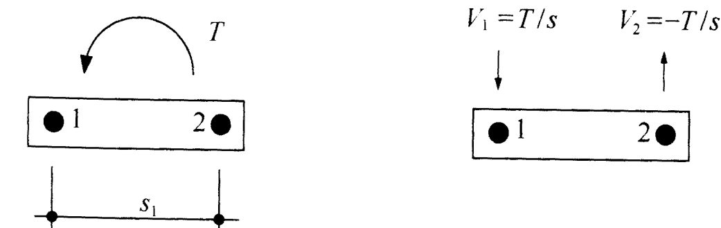
(a) 作用在群锚上的扭矩
