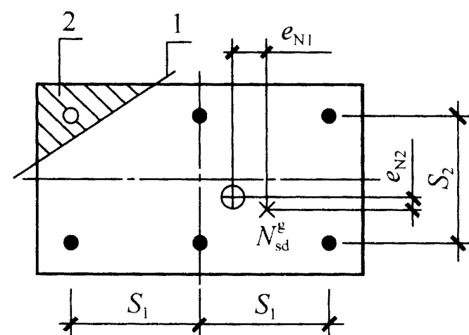
图 5.2.4-3 群锚双向偏心受拉示意
