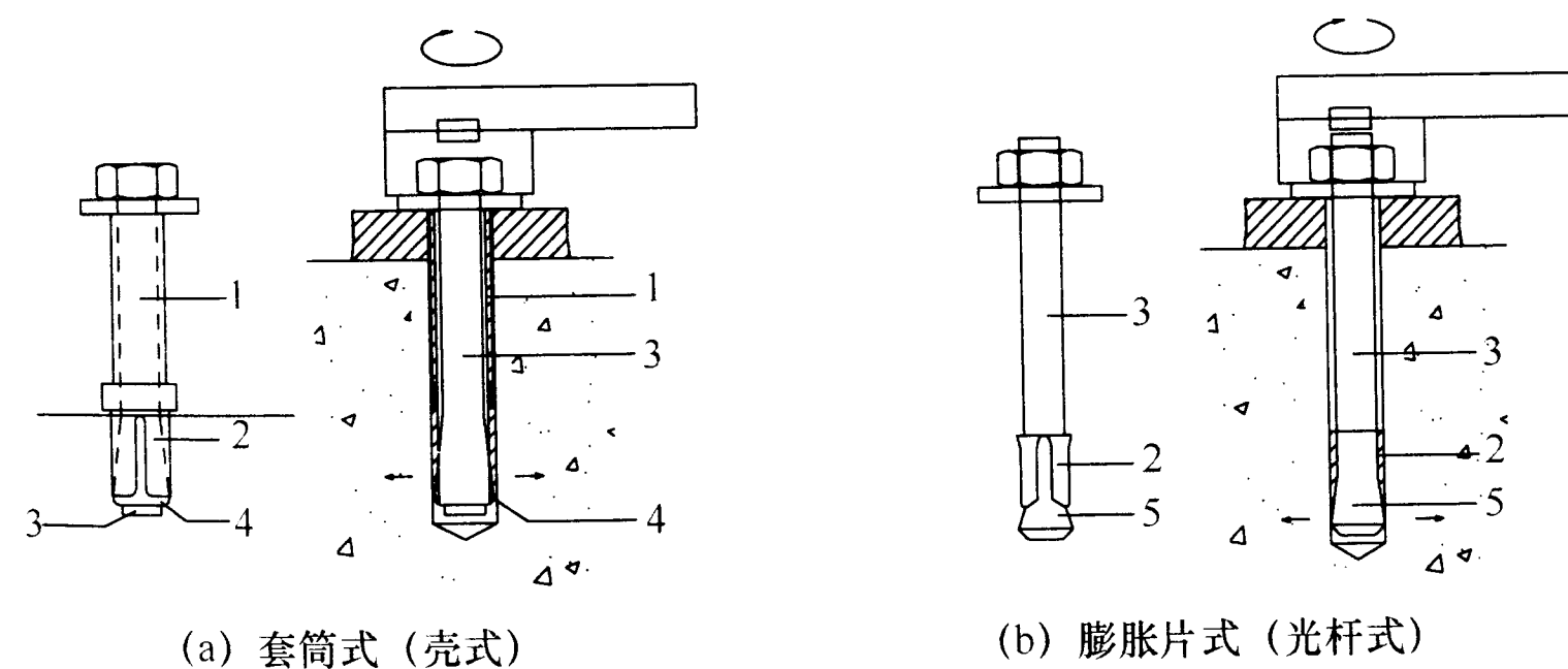
图 A.1.2-1 扭矩控制式膨胀型锚栓示意
