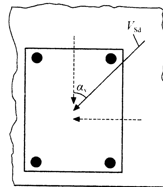
图 6.1.21 剪力角 \alpha_v 示意
