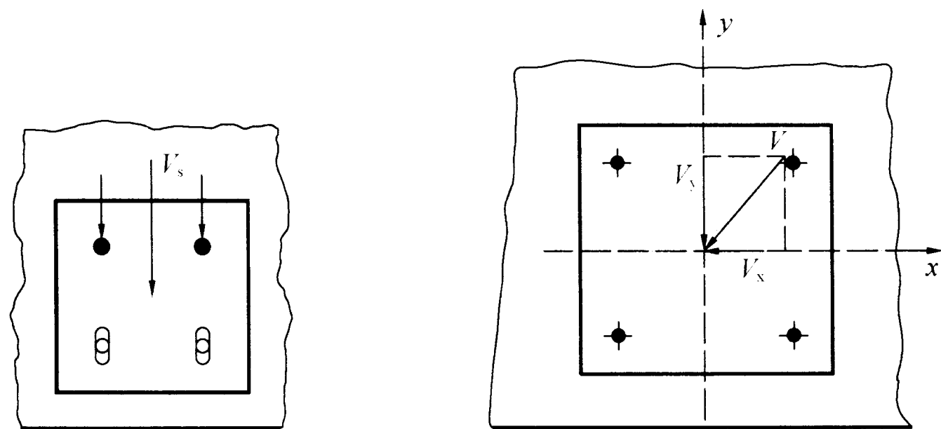
图 5.3.2 长槽孔处锚栓 不承担剪力示意
