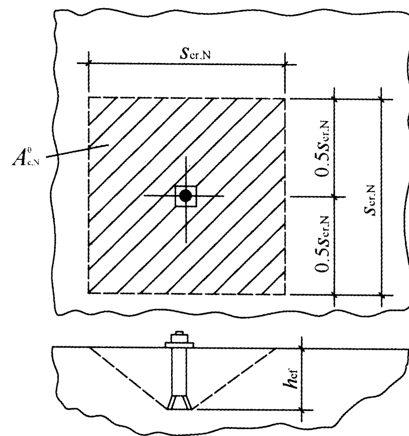
图 6.1.4 理想锥体破坏投影面面积示意
