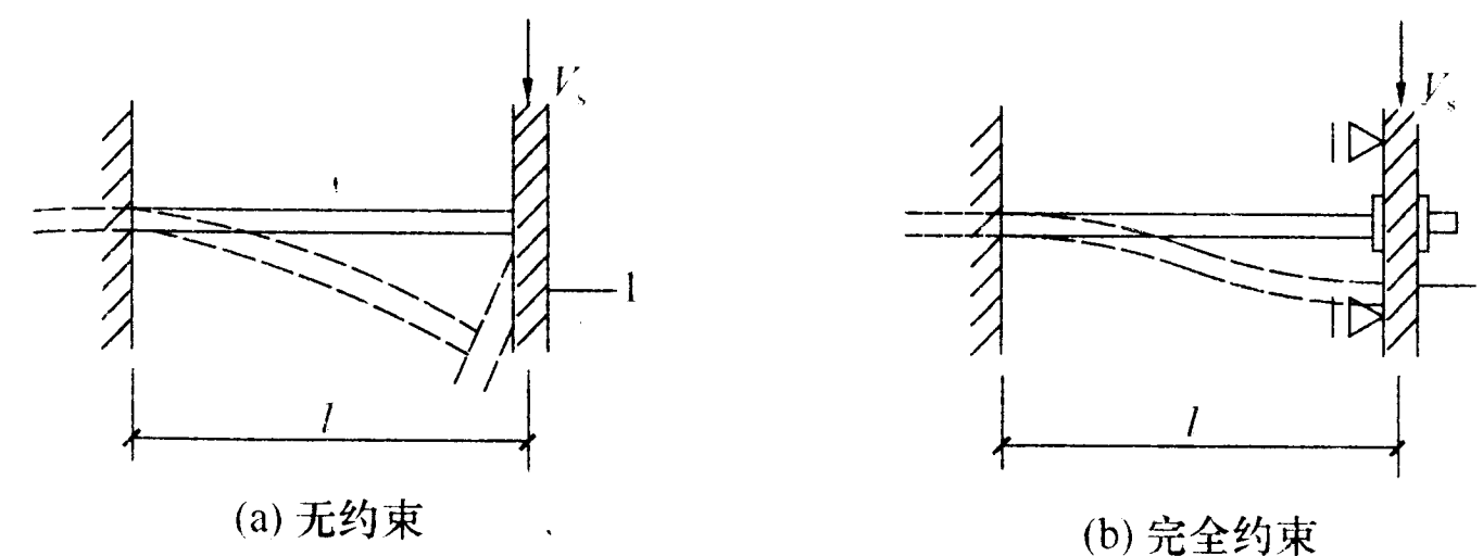
图 6.1.14-2 约束状况示意
