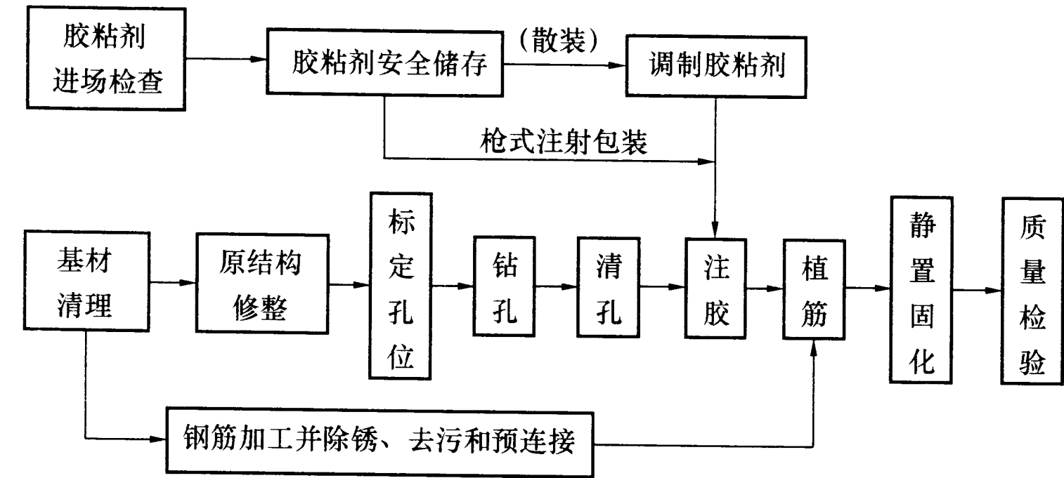
图 6 植筋施工工序示意
