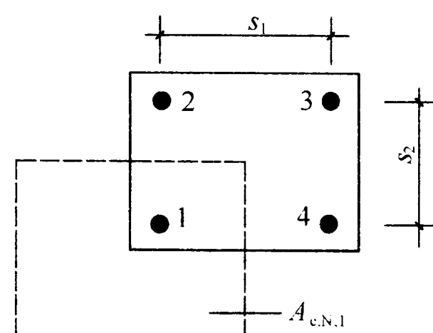
图 6.1.27-3 四栓, 无边距影响示意
