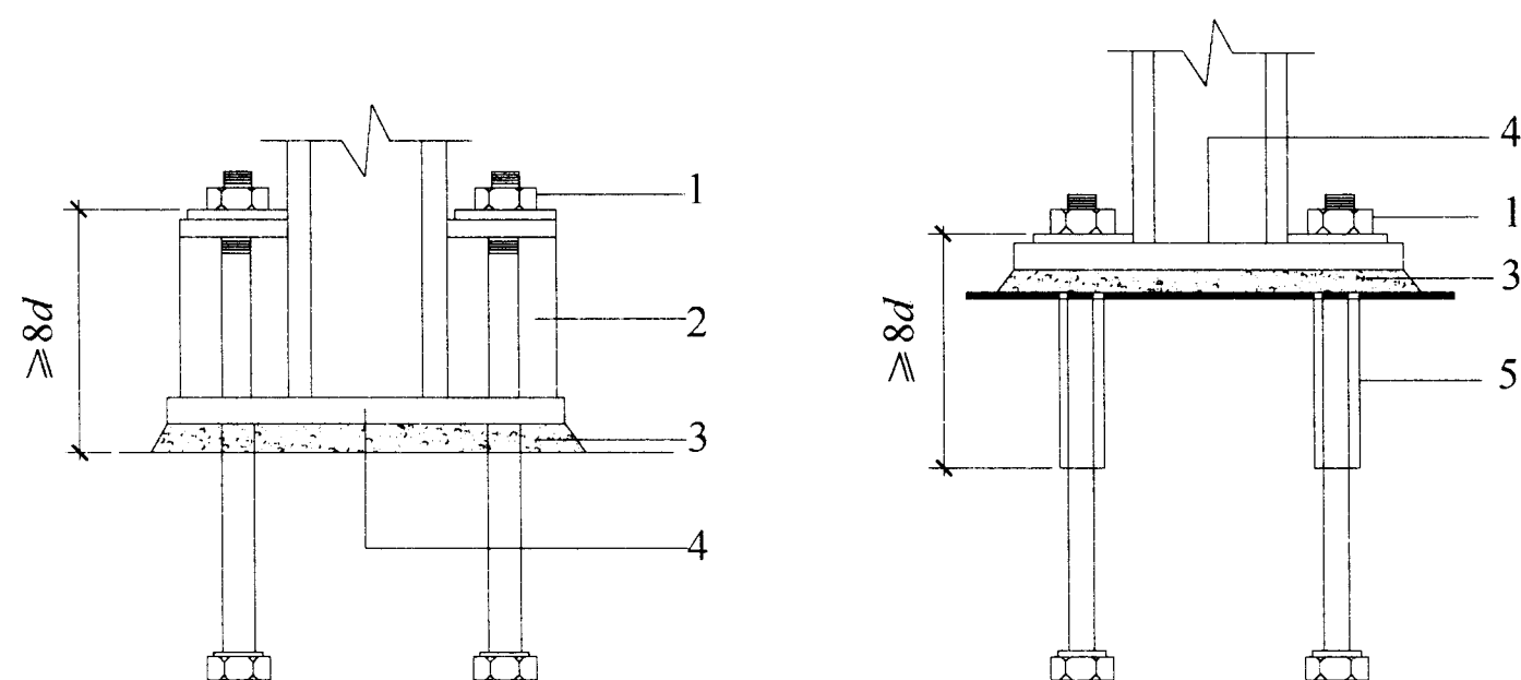
图 8.2.2 锚栓延性伸长段示意图
