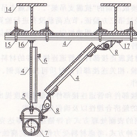
(h) 钢结构单侧向抗震支吊架构造形式
