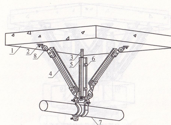
(b) 单管双向抗震支吊架构造形式
