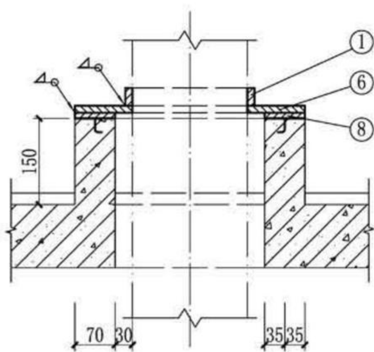
图3 (预埋件固定)
