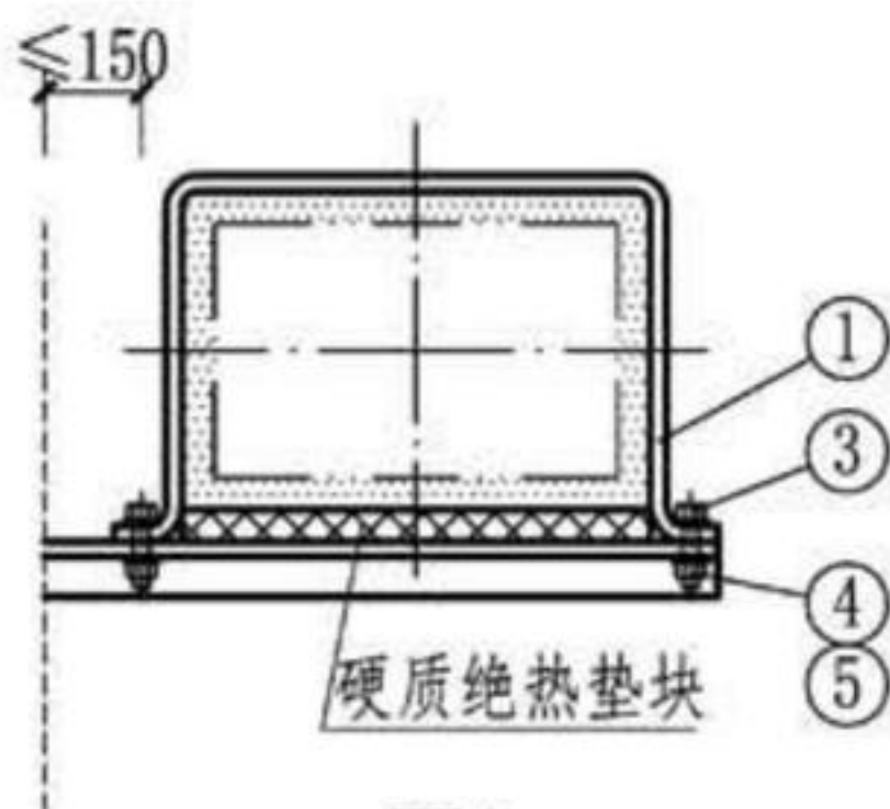
图4 (保温、扁钢管卡、螺栓固定)
