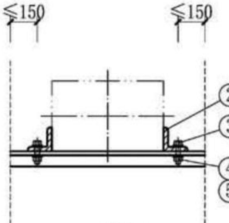
图7 (无保温、角钢管卡、螺栓固定)
