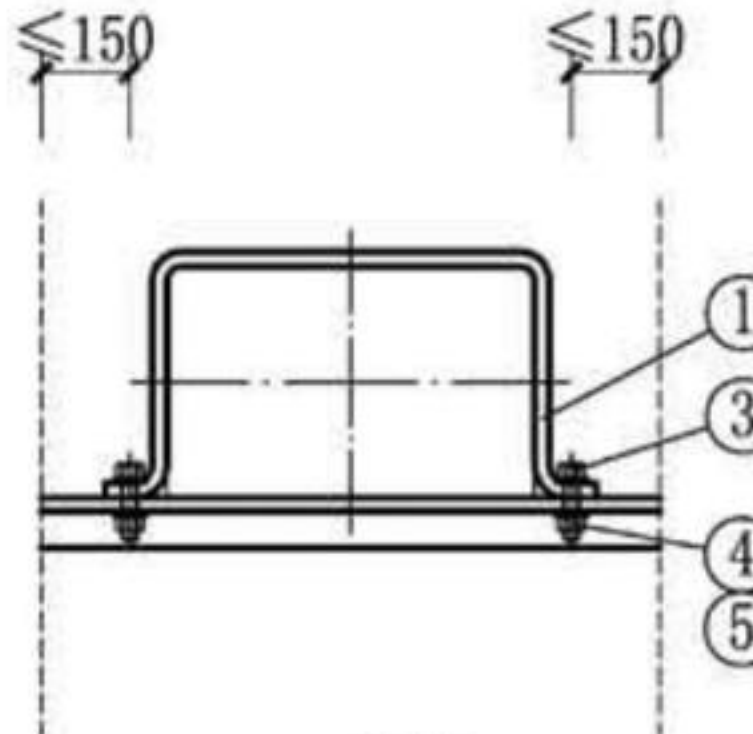
图6 (无保温、扁钢管卡、螺栓固定)
