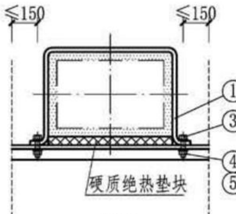
图9 (保温、扁钢管卡、螺栓固定)
