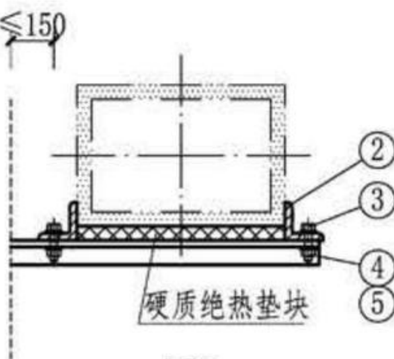
图5 (保温、角钢管卡、螺栓固定)
