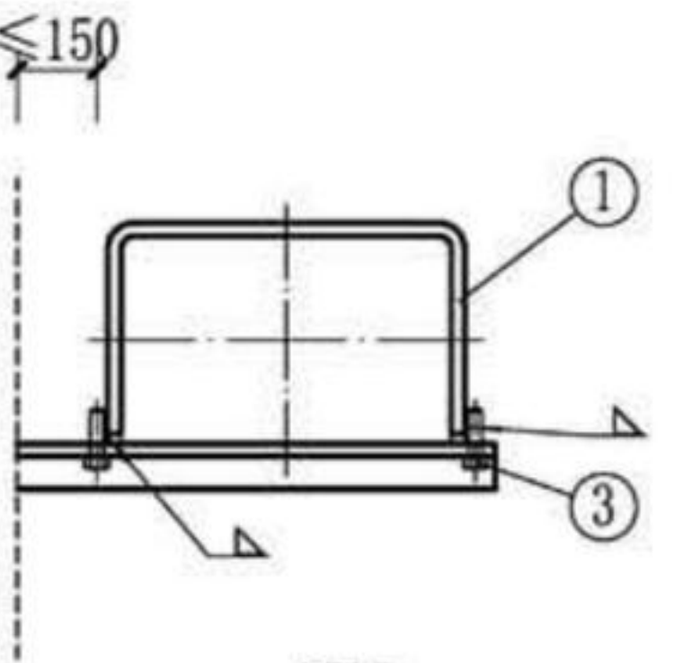
图3 (无保温、扁钢管卡、螺栓固定)
