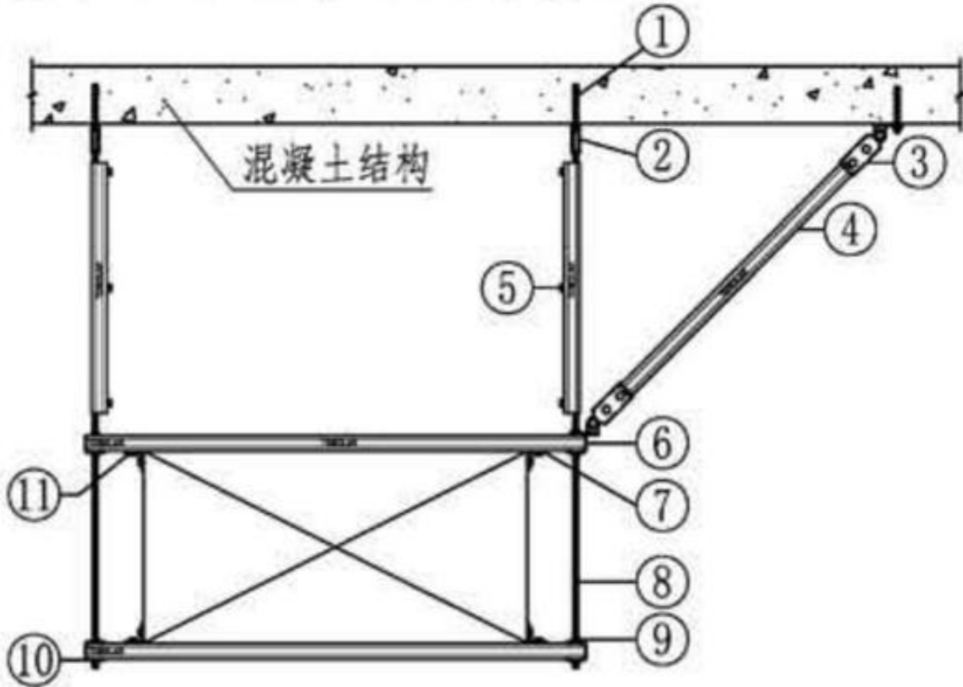
通风管道四向抗震支架
