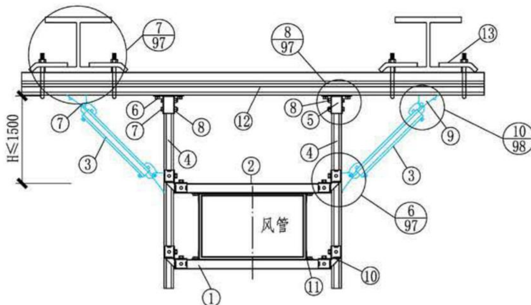
矩形风管双侧向抗震支吊架正视图
