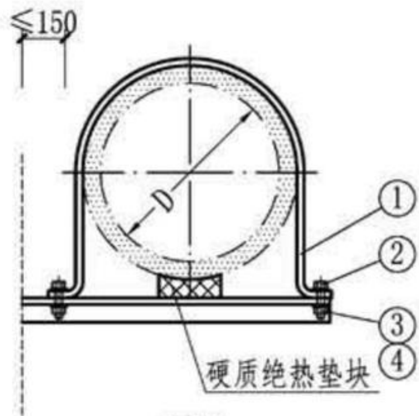
图1 (螺栓螺母固定)
