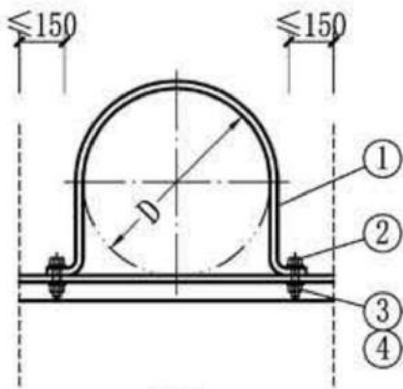
图4 (螺栓螺母固定)
