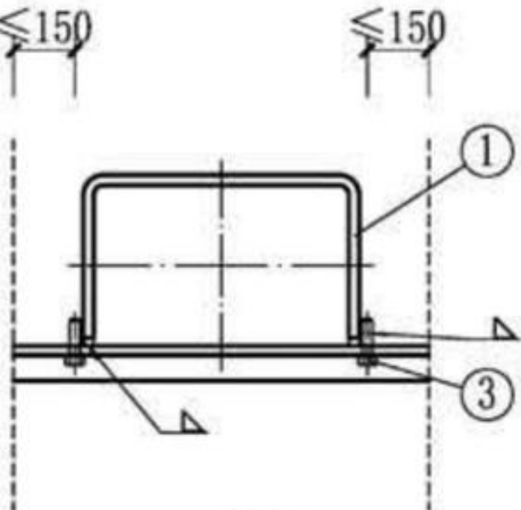
图8 (无保温、扁钢管卡、螺栓固定)
