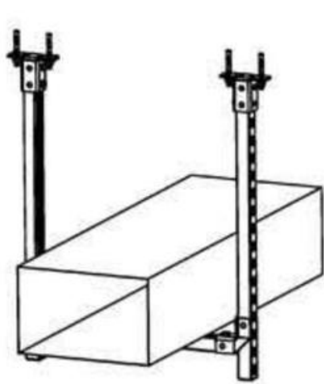
矩形风管刚性支吊架
