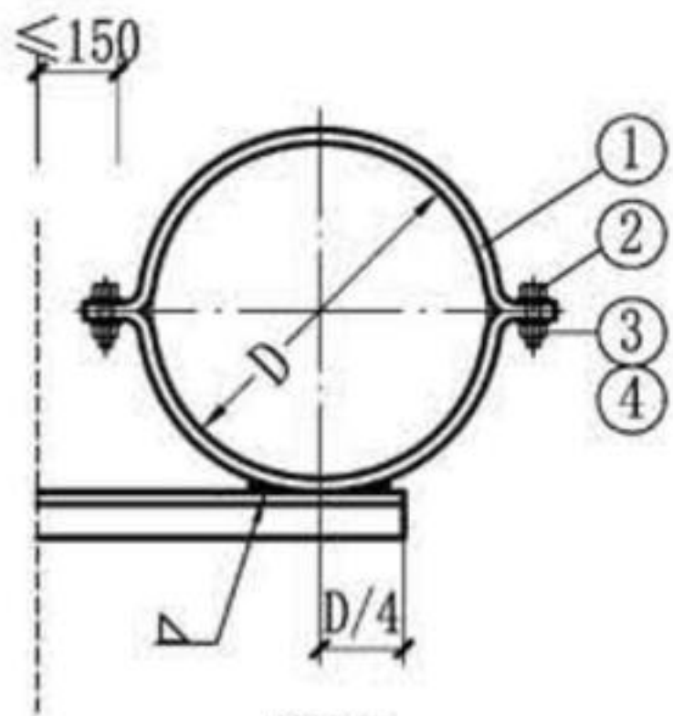
图3 (焊接固定)
