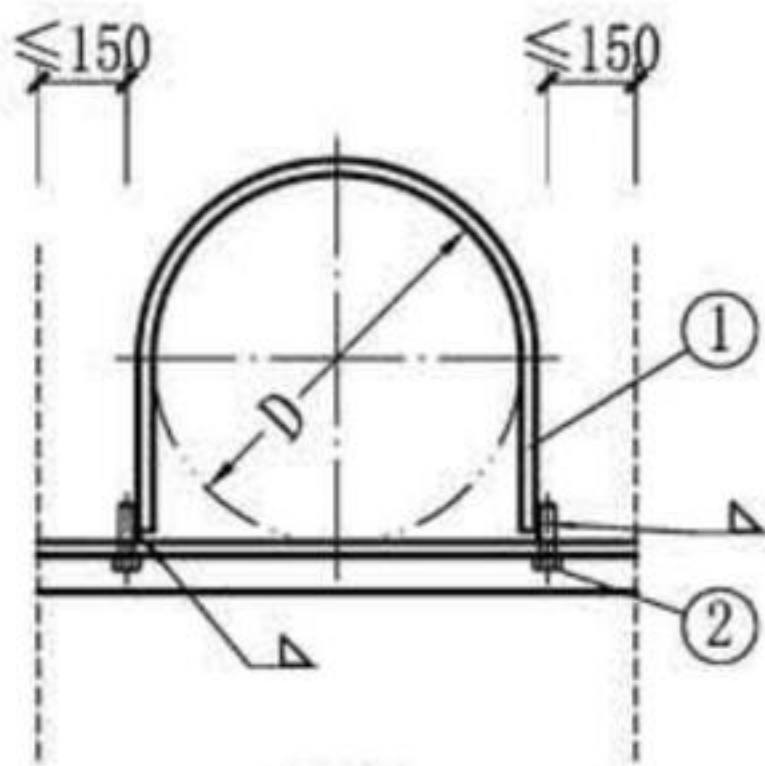
图5 (螺栓焊接固定)
