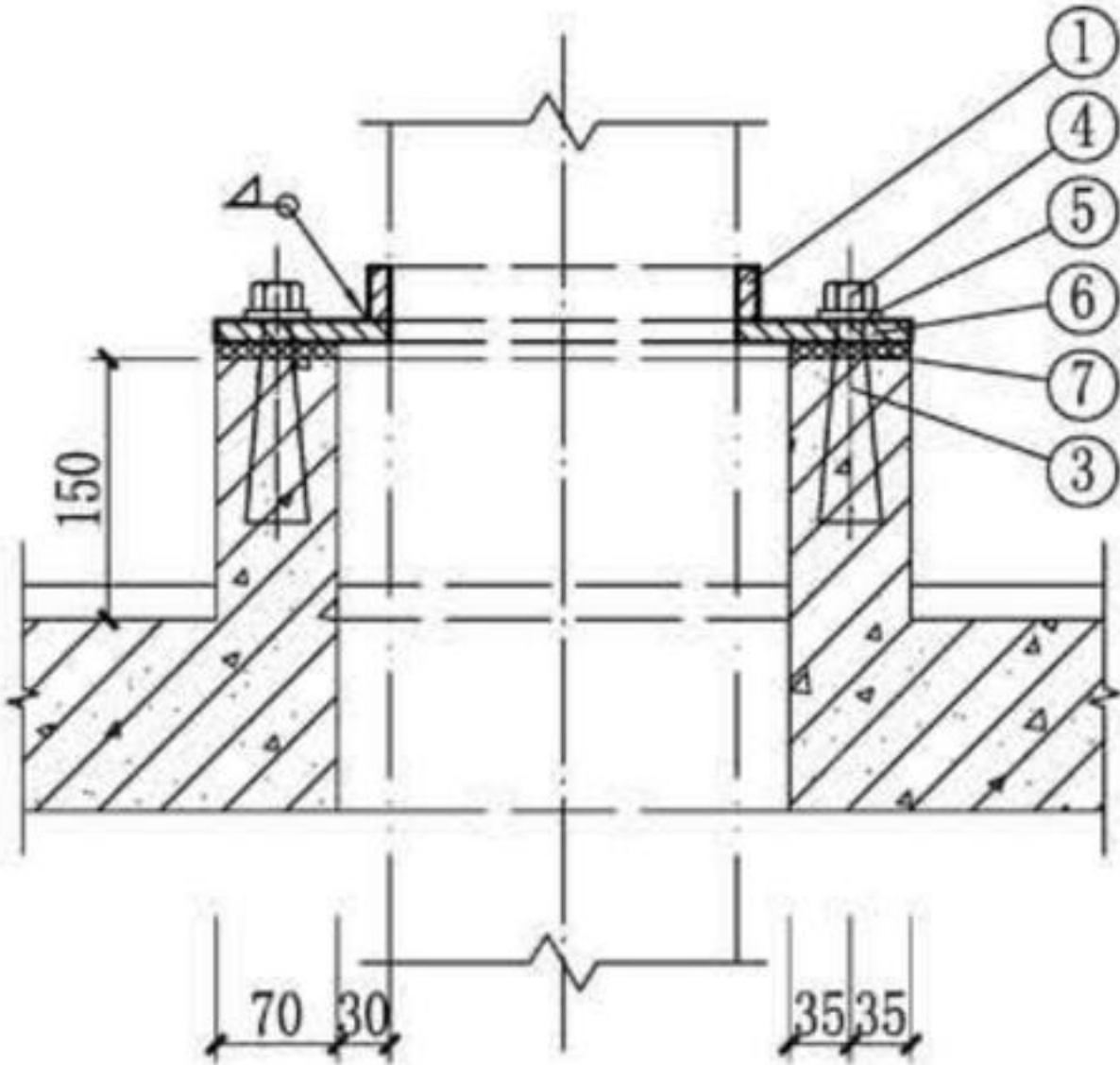
图2 (膨胀型锚栓固定)
