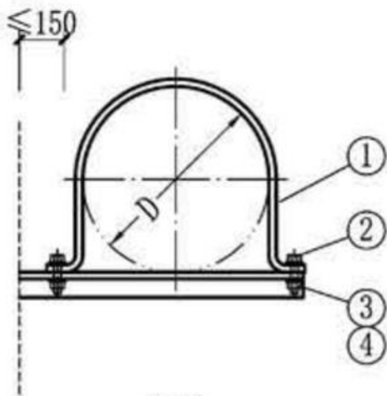
图1 (螺栓螺母固定)
