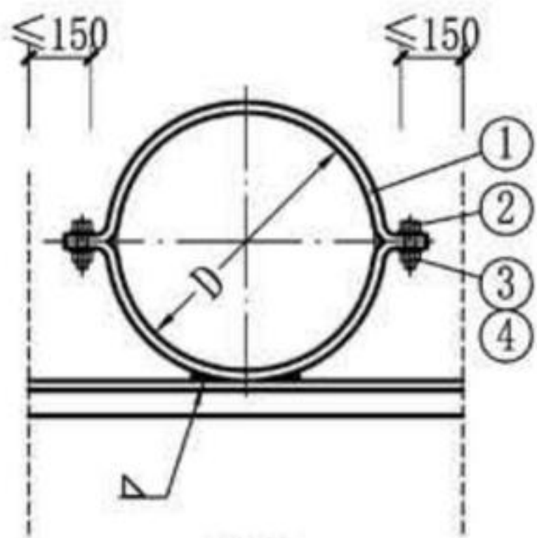
图6 (焊接固定)
