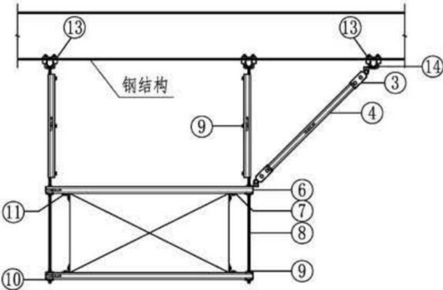
通风管道侧向抗震支架
