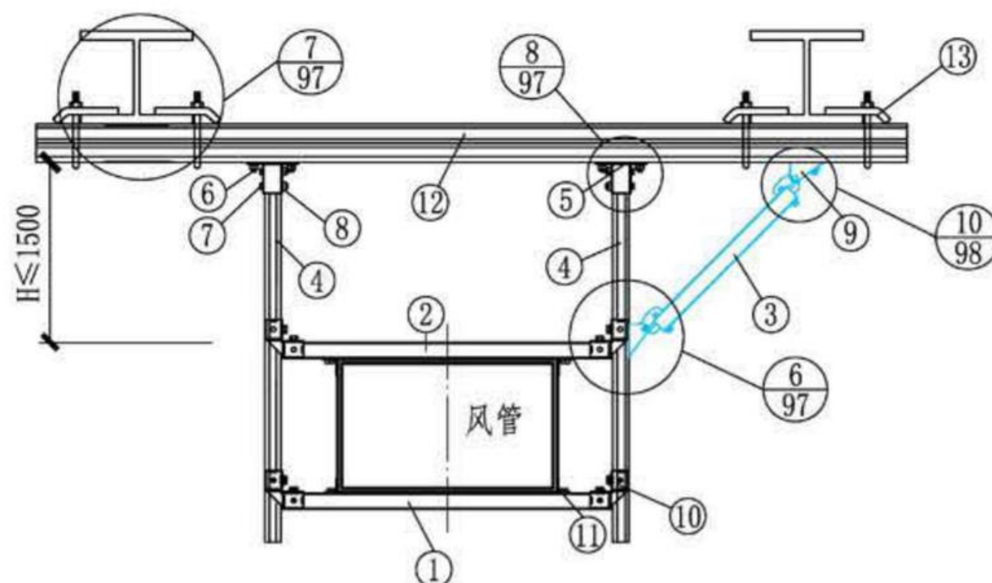
矩形风管单侧向抗震支吊架正视图
