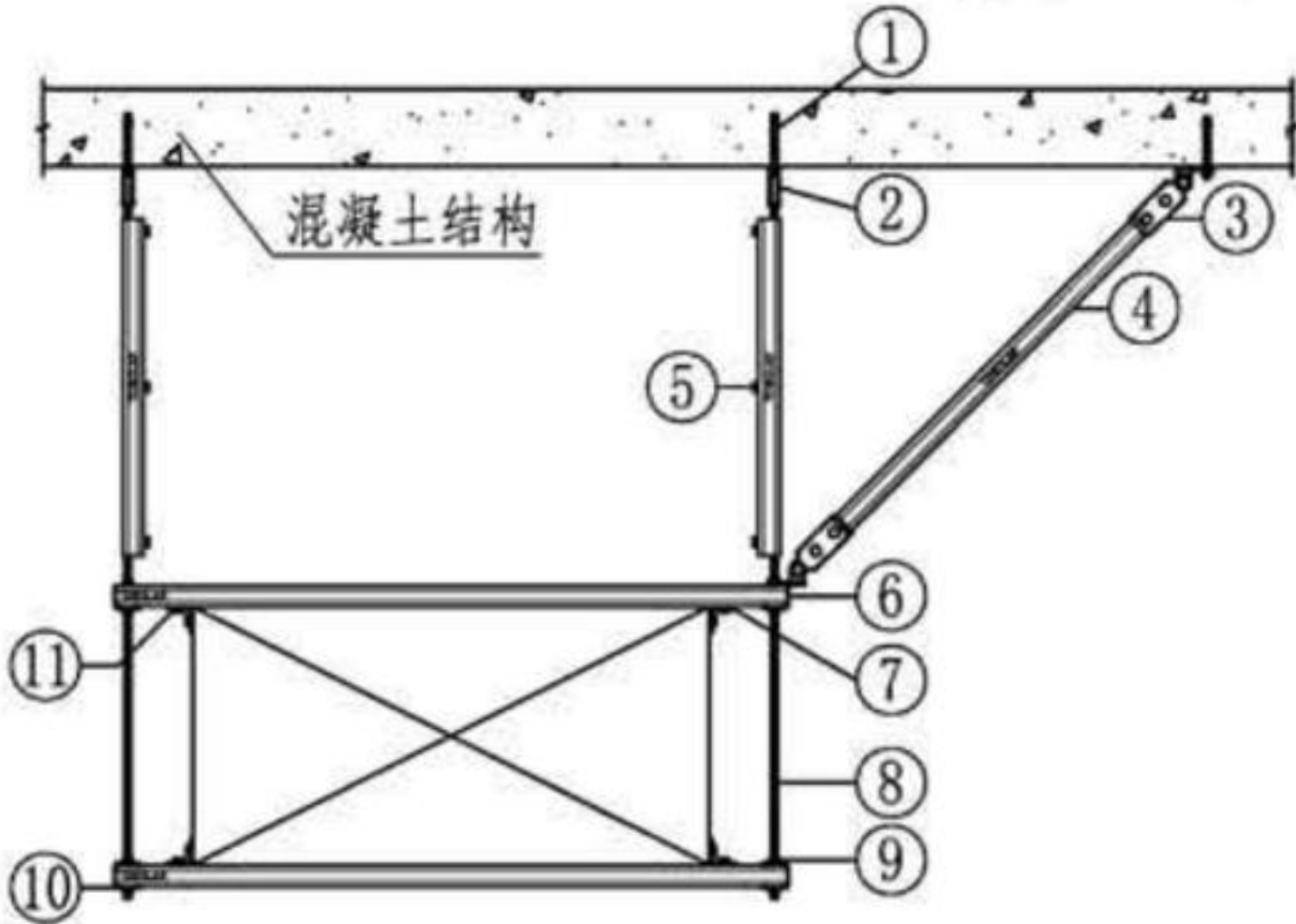
通风管道侧向抗震支架
