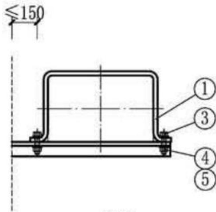
图1 (无保温、扁钢管卡、螺栓固定)
