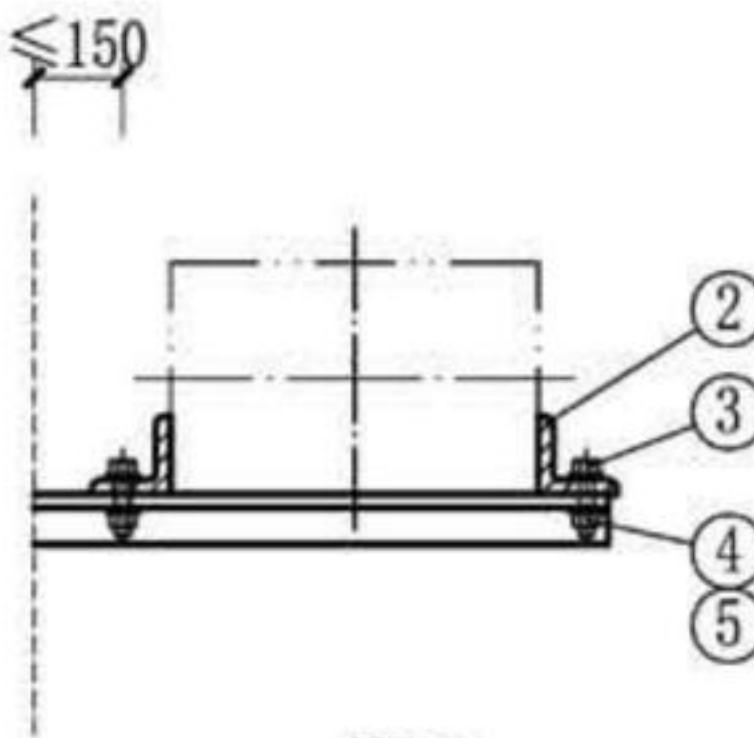
图2 (无保温、角钢管卡、螺栓固定)
