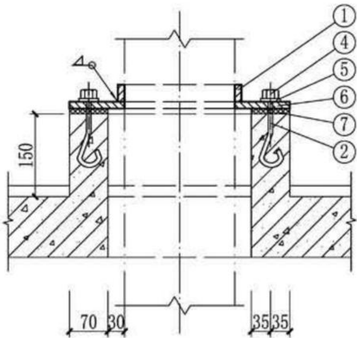
图1 (地脚螺栓固定)
