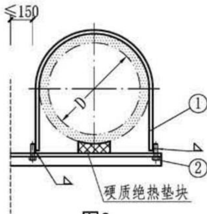
图2 (螺栓焊接固定)
