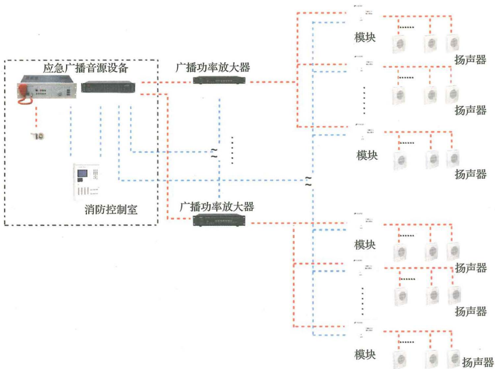
图 12-4 消防应急广播系统构成示意图
