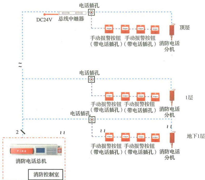
图 12-5 消防电话系统构成示意图
