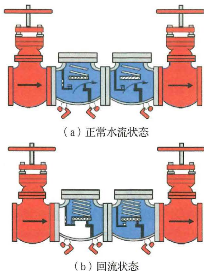
图 3-4 双止回阀倒流防止器
