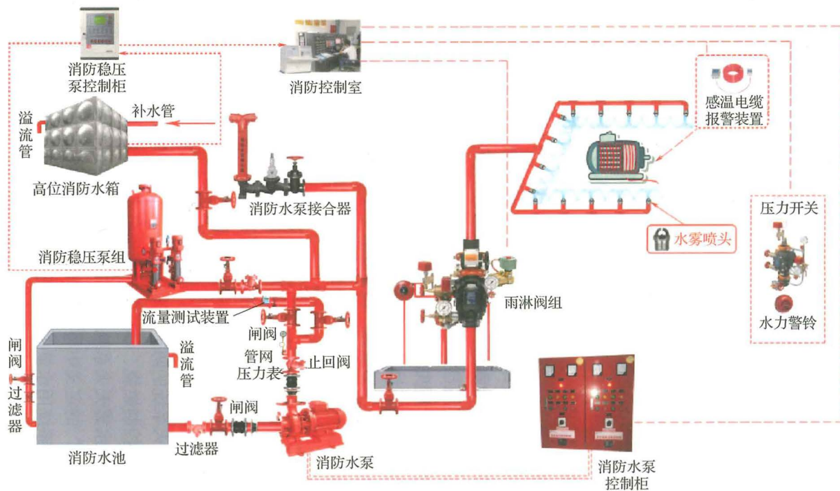
图 6-1 水喷雾灭火系统构成示意图
