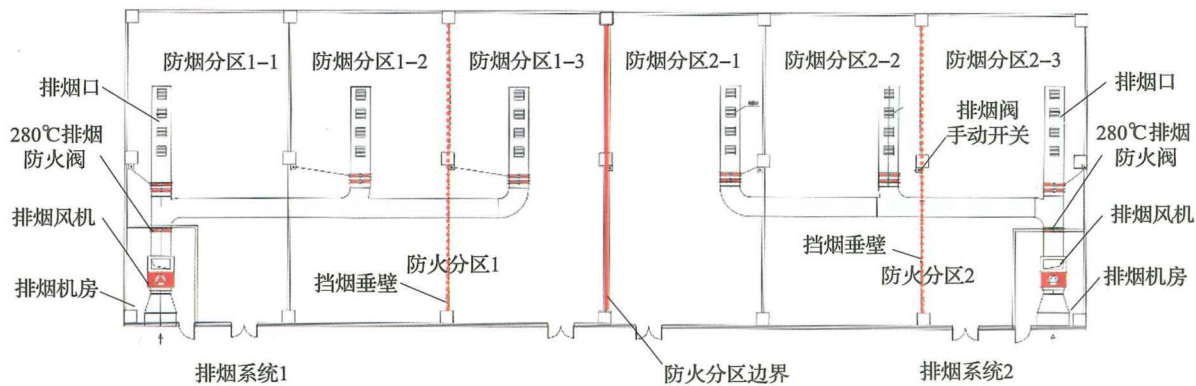
图 11-6 机械排烟系统横向布置示意图
