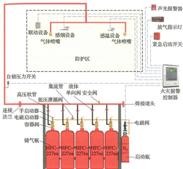
图 8-1 管网式气体灭火系统构成示意图
