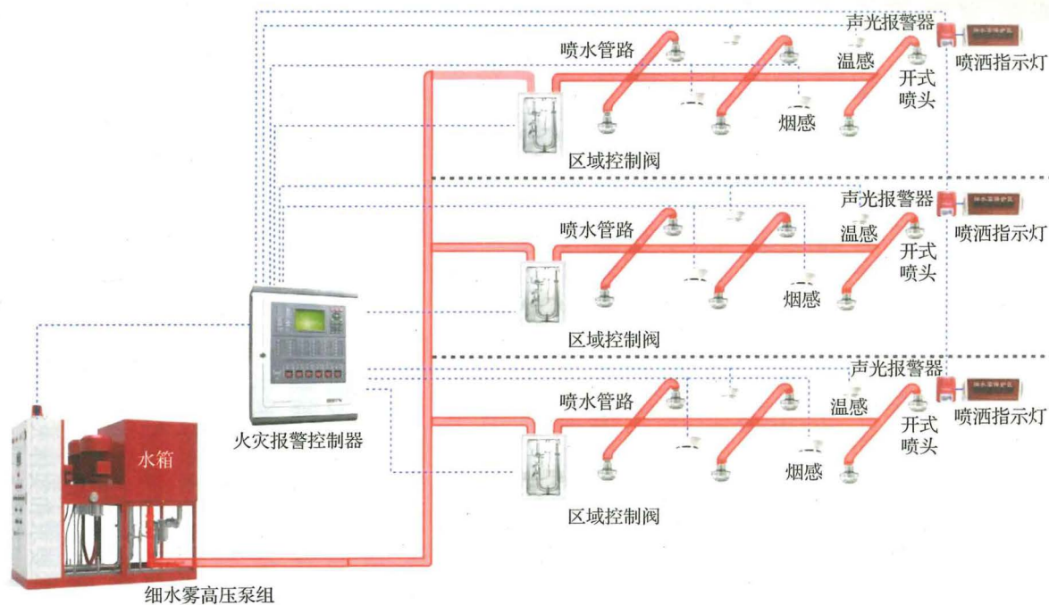
图 6-2 细水雾灭火系统构成示意图
