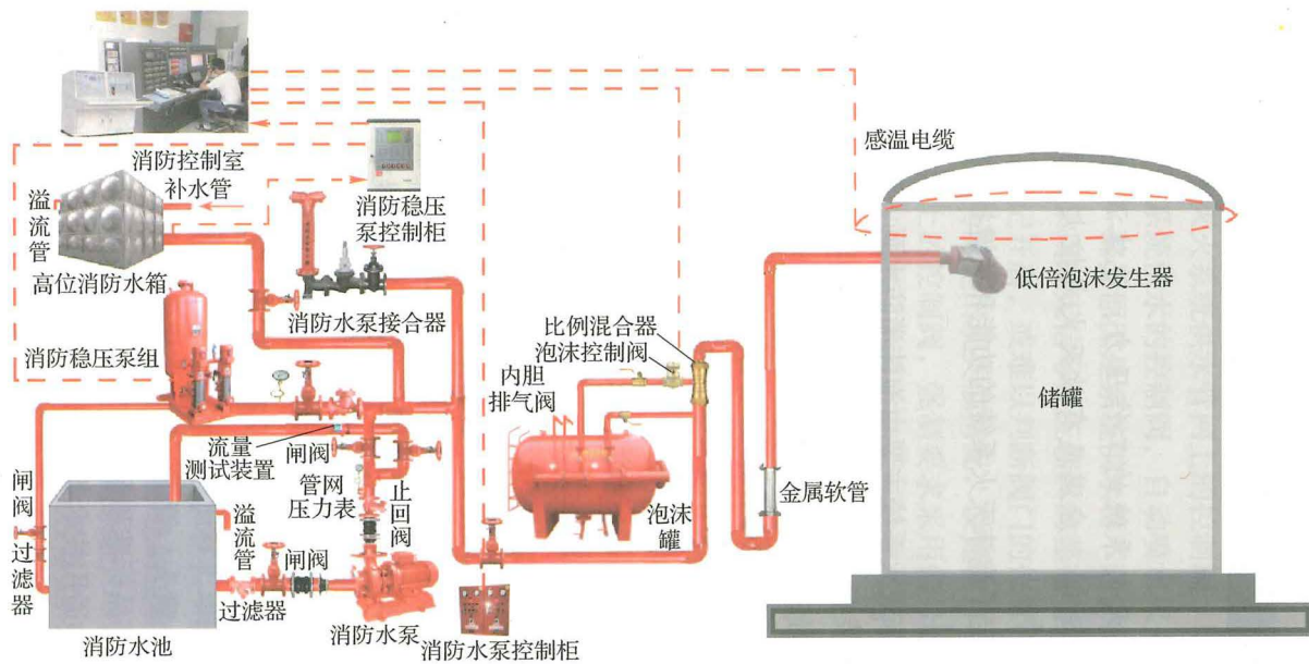
图 5-1 低倍泡沫灭火系统构成示意图
