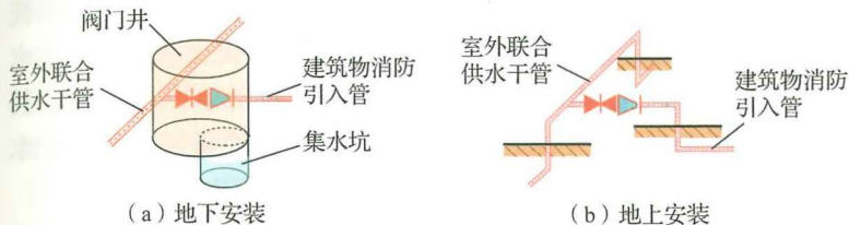
图 3-8 减压型倒流防止器安装示意图
