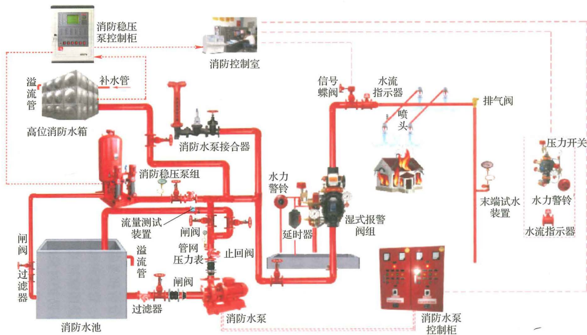
图 4-1 湿式自动喷水灭火系统构成示意图
