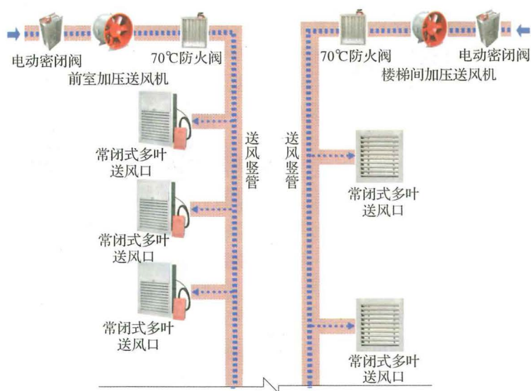
图 11-1 机械加压送风系统构成示意图
