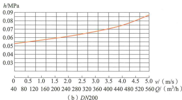
图 3-6 减压型倒流防止器的水头损失曲线
