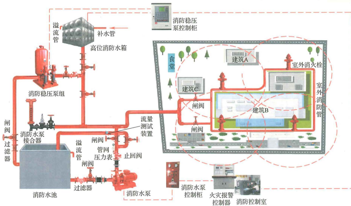
图 3-3 室外消火栓系统构成示意图
