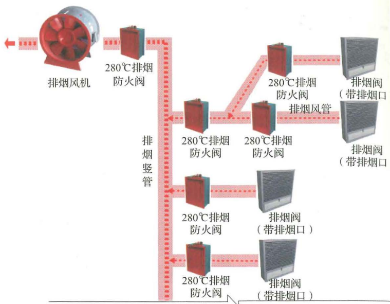
图 11-2 机械排烟系统构成示意图
