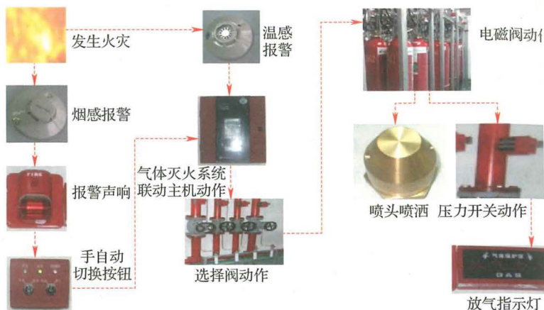
图 8-4 气体灭火系统联动控制自动启动示意图
