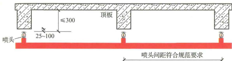
图 4-2 梁下直接布置喷头的情况
