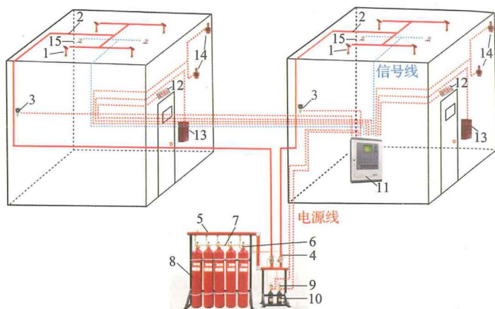
1—喷嘴；2—管道；3—压力信号器；4—选择阀；5—集流管；6—容器阀；7—单向阀； 8—储存容器；9—启动装置；10—氮气瓶；11—火灾报警控制器；12—放气指示灯； 13—紧急启停按钮；14—声光报警器；15—火灾探测器。
