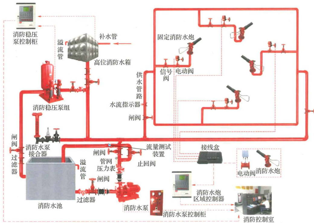
图 7-1 固定消防炮灭火系统构成示意图
