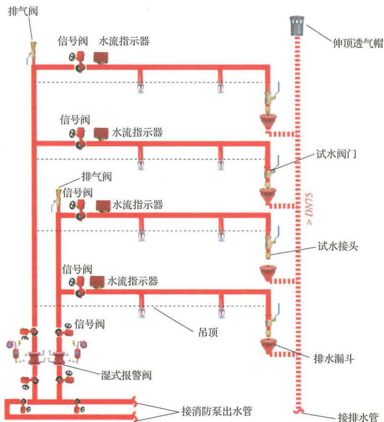
图 4-5 末端试水装置和试水阀设置示意图
