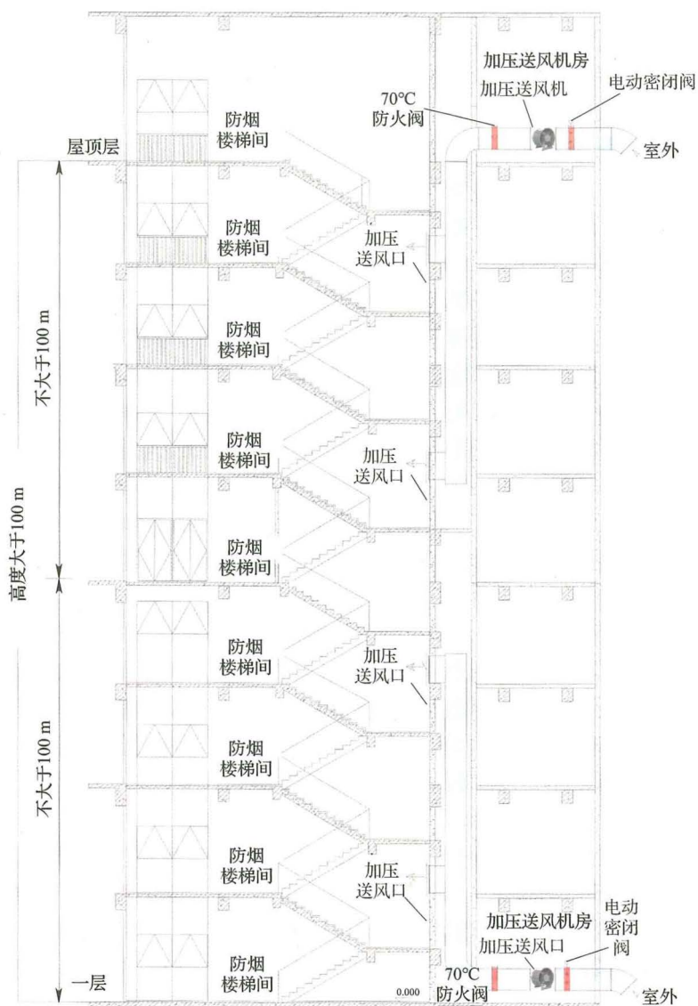
图 11-4 楼梯间内的机械加压送风系统分段设置示意图
