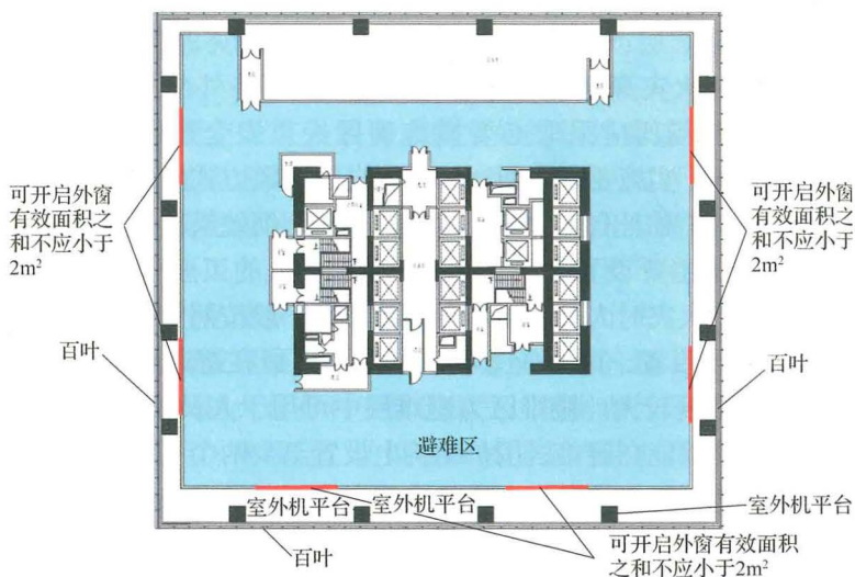
图 11-5 避难层自然通风口设置示意图
