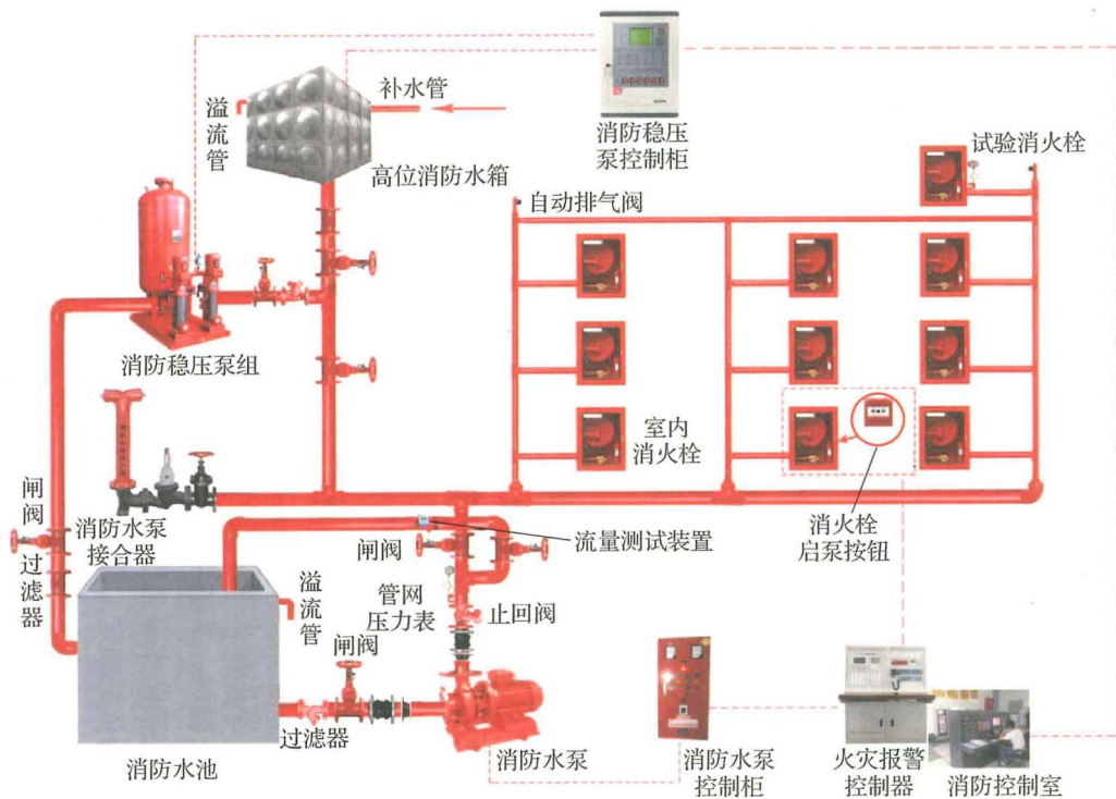
图 3-7 室内消火栓系统构成示意图
