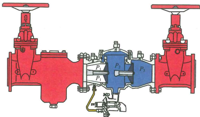
图 3-5 减压型倒流防止器
