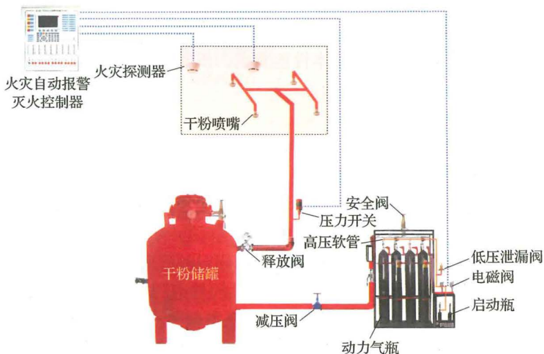
图 9-1 全淹没干粉灭火系统的构成示意图
