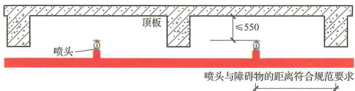
图 4-3 梁间布置喷头的情况
