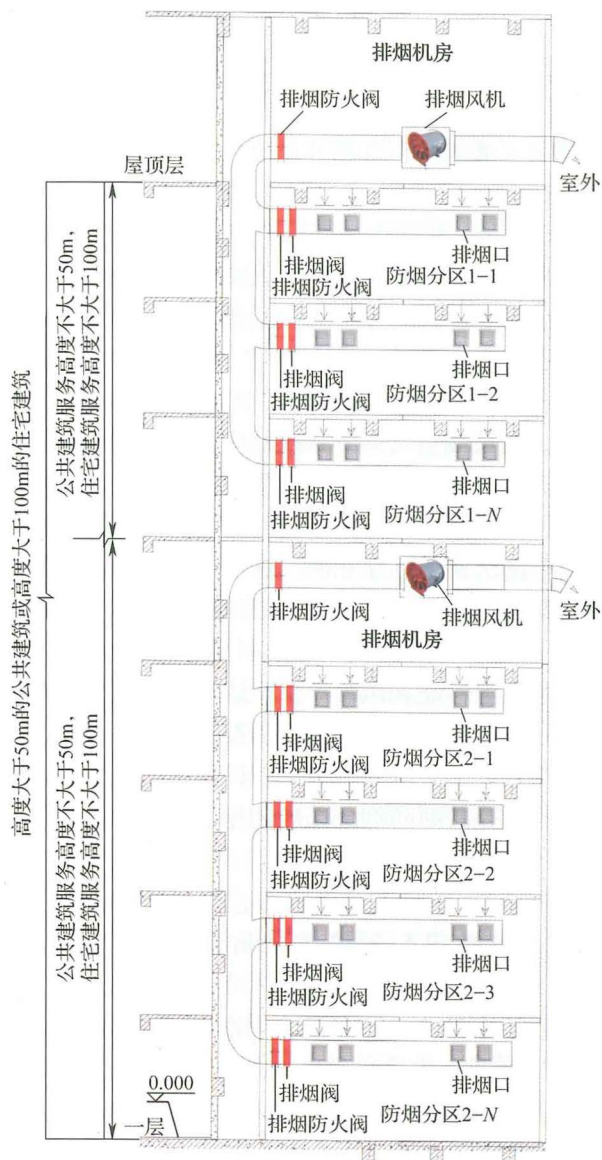
图 11-7 机械排烟系统竖向分段布置示意图
