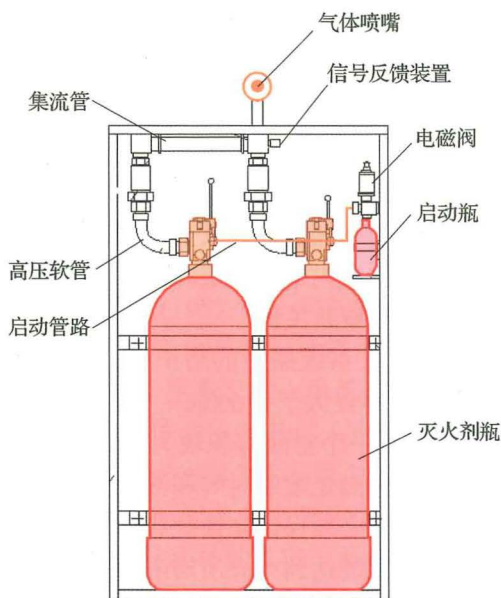
图 8-3 无管网式预制气体灭火系统构成示意图
