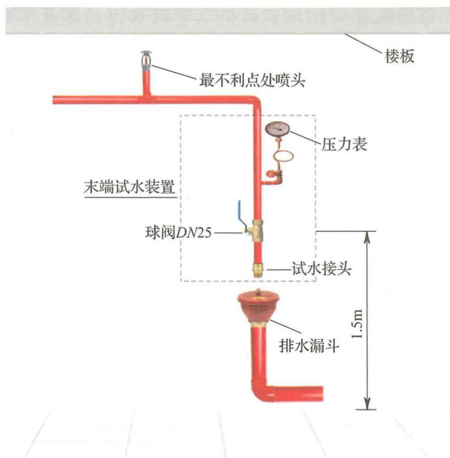
图 4-4 末端试水装置布置示意图
