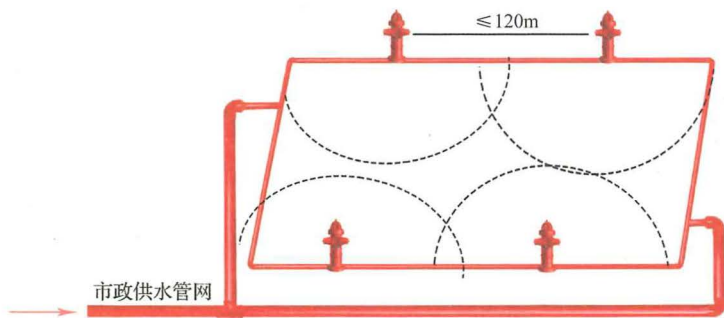
图 3-2 市政消火栓系统构成示意图
