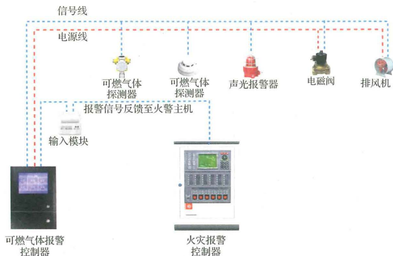
图 12-6 可燃气体探测报警系统构成示意图
