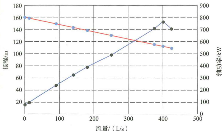
图 3-1 消防水泵流量扬程曲线图
