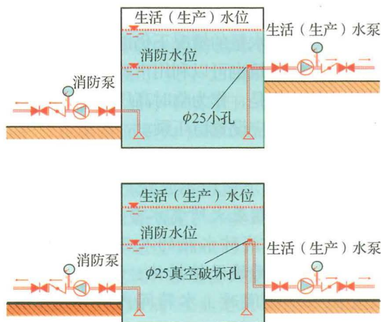
图 3-9 合用水池消防用水报警水位
